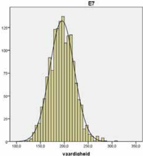
Figuur 3.2 Weergave van behaalde vaardigheidsscores met bijbehorende normale verdeling voor afnamemoment E7
