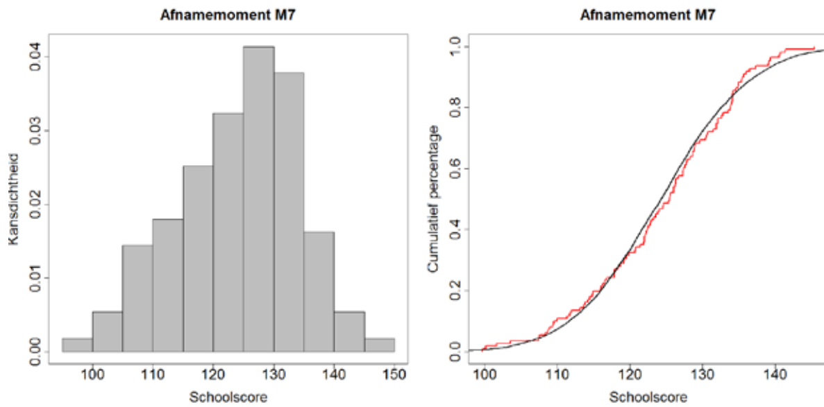
Figuur 4.7 Verdeling van de schoolgemiddelden voor LVS 3.0 Begrijpend lezen M7
