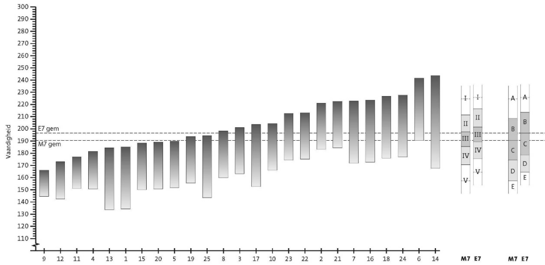
Moeilijkheid van opgaven M7 - Taak 1
