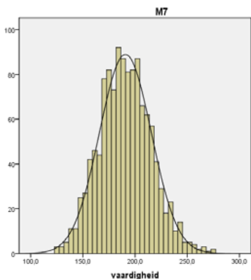
Figuur 3.1 Weergave van behaalde vaardigheidsscores met bijbehorende normale verdeling voor afnamemoment M7
