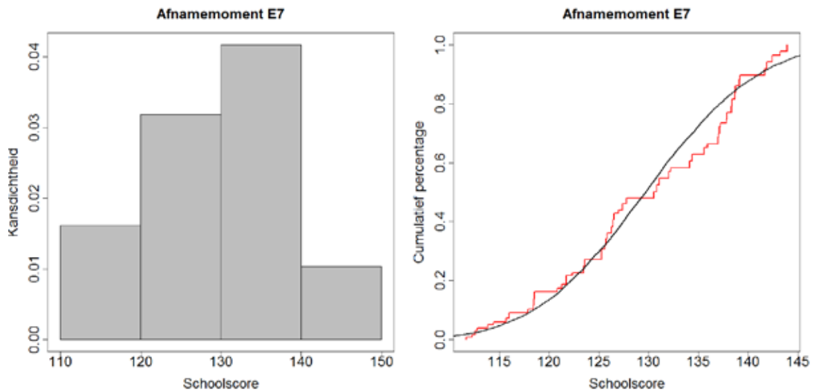
Figuur 4.8 Verdeling van de schoolgemiddelden voor LVS 3.0 Begrijpend lezen E7
