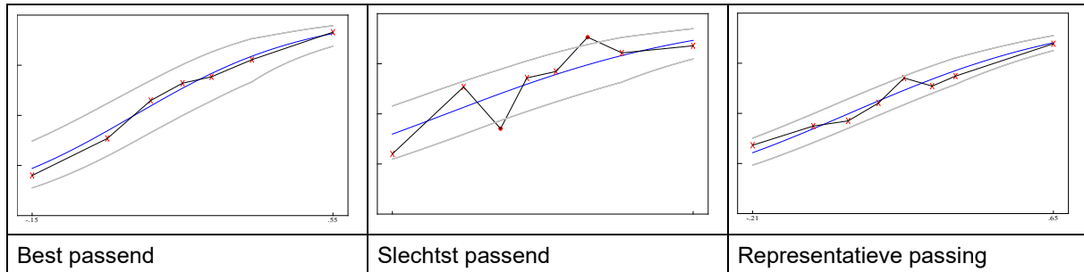
Figuur 4.6 Voorbeelden van S-toetsen voor de Toets LVS 3.0 Begrijpend lezen M7 en E7 met de best passende, de slechtst passende en een qua passing representatieve opgave
