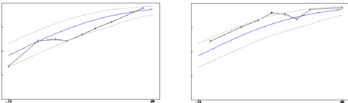
Figuur 6.1 Item-bias met betrekking tot sekse
