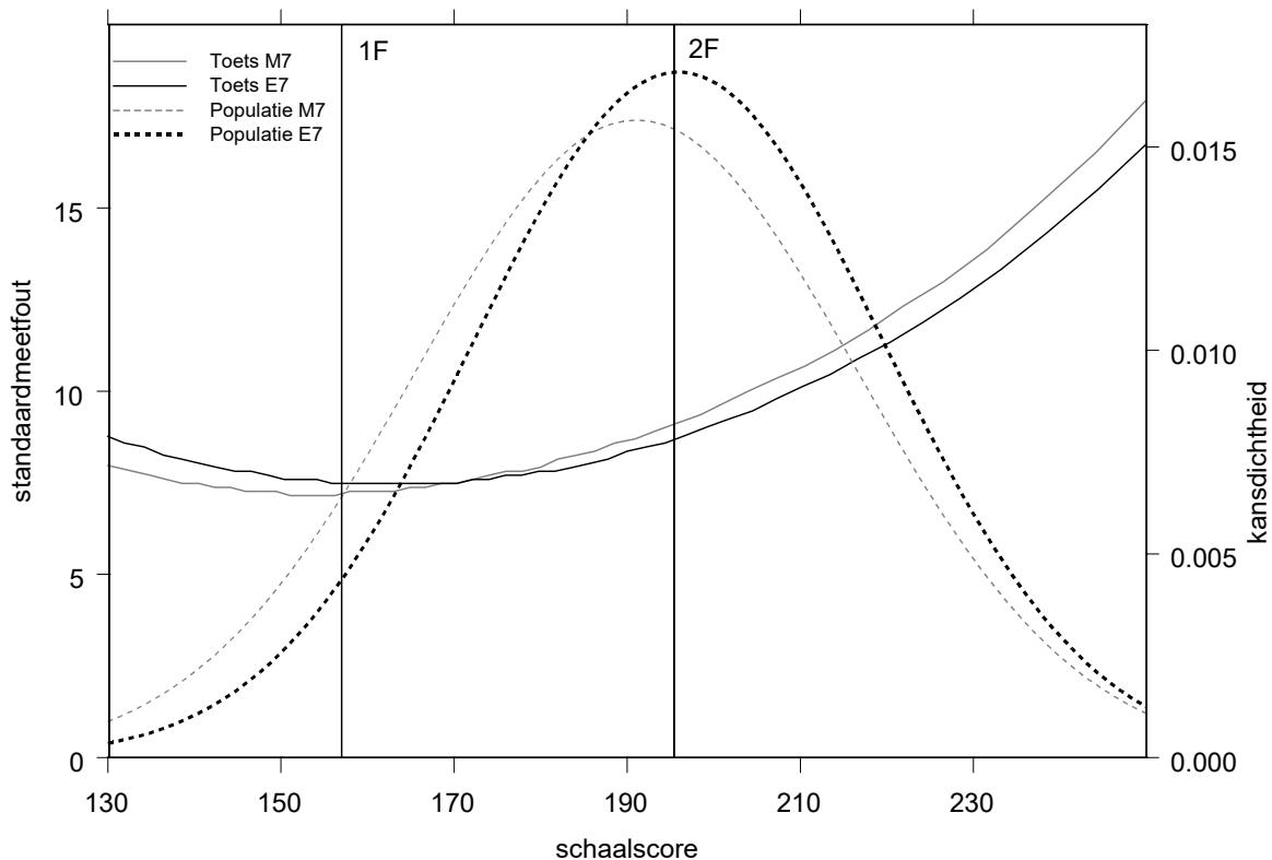
Figuur 5.1 Grootte van de meetfouten voor de toetsen M7 en E7 en de bijbehorende kansdichtheidsfuncties
