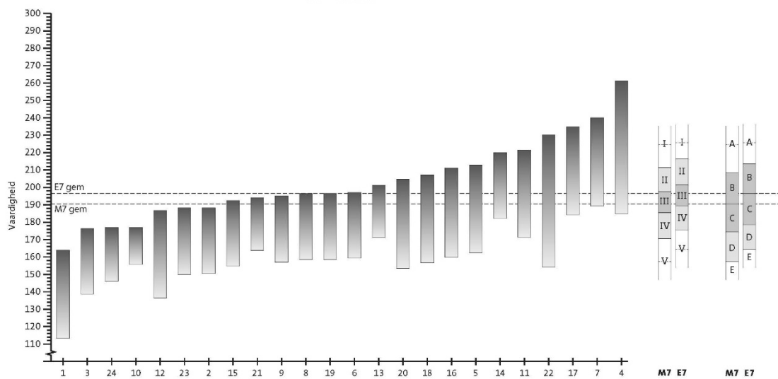
Moeilijkheid van opgaven M7 - Taak 2
