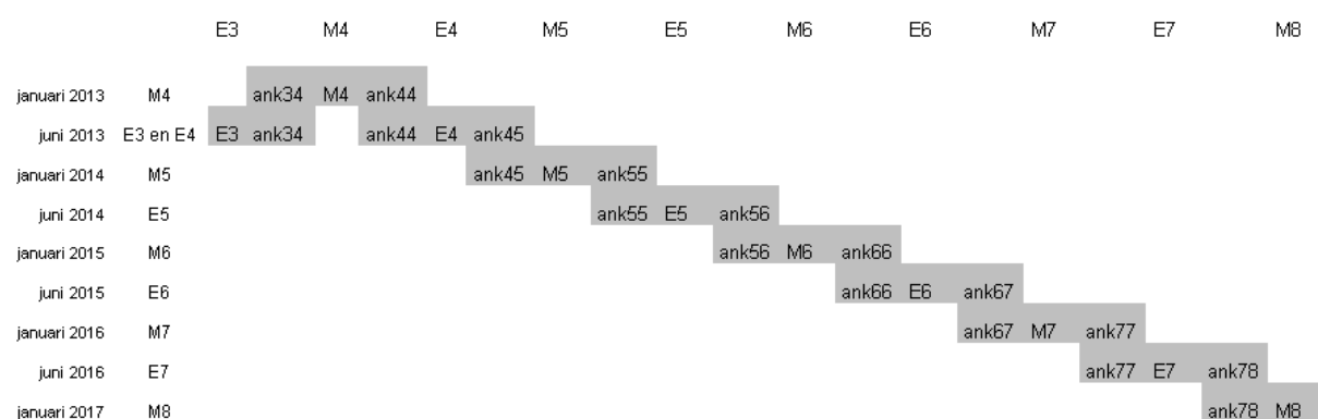
Figuur 4.1 Macrodesign LVS 3.0 Begrijpend lezen
